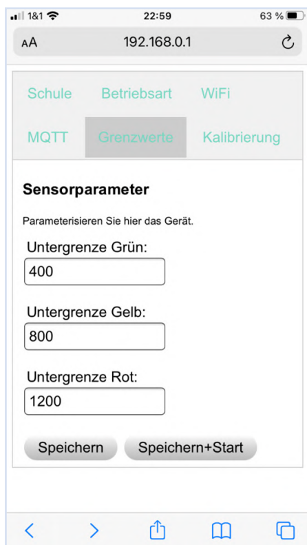
Figure 4. Une des pages web de configuration. Les utilisateurs peuvent saisir les seuils pour le feu tricolore. Une version anglaise des pages web est prévue.
