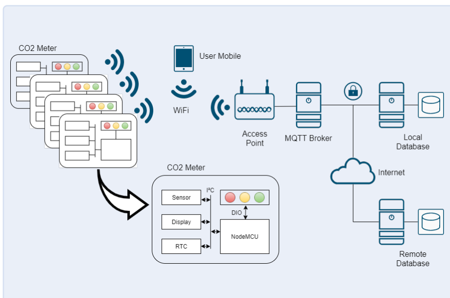
Figure 3. Nos compteurs de CO 2 peuvent envoyer leurs données au réseau via le protocole MQTT [8].
