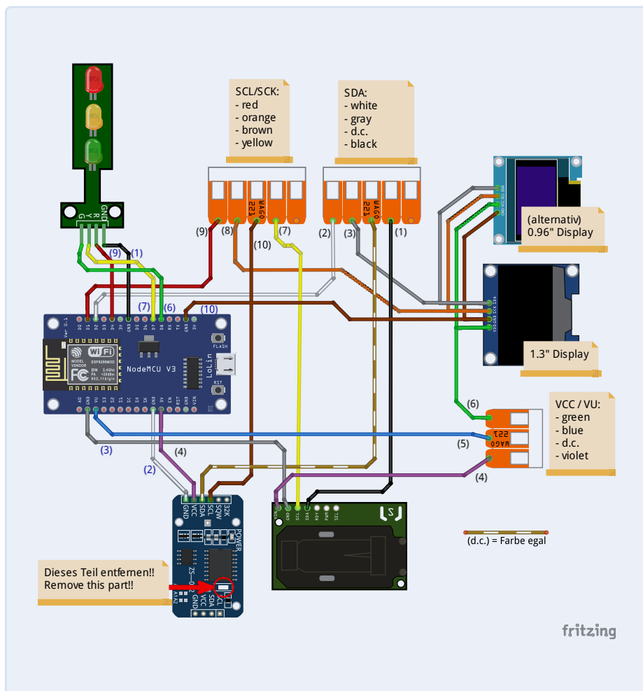
Figure 2. Schéma Fritzing des modules, avec l'ESP8266 comme cerveau du projet.
