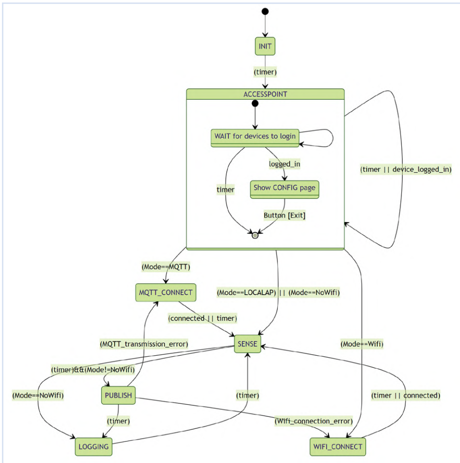
Figure 8. Automate fini implémenté dans le logiciel.
