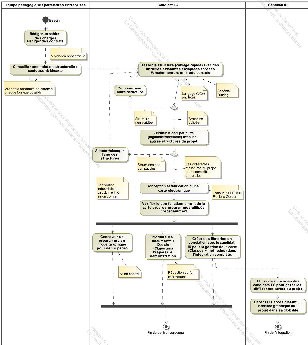
Diagramme d'activités : du point de vue Électronique et Communications
