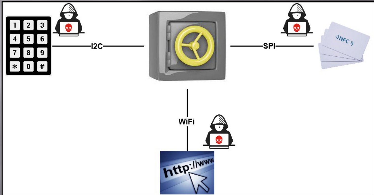
Synoptique général
